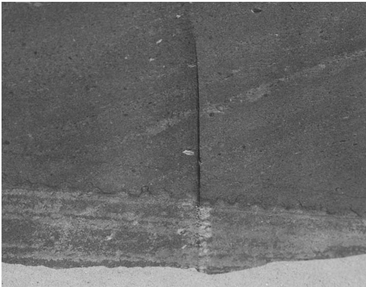
Рис. 16. След от дисковой пилы на блоке черного базальта
