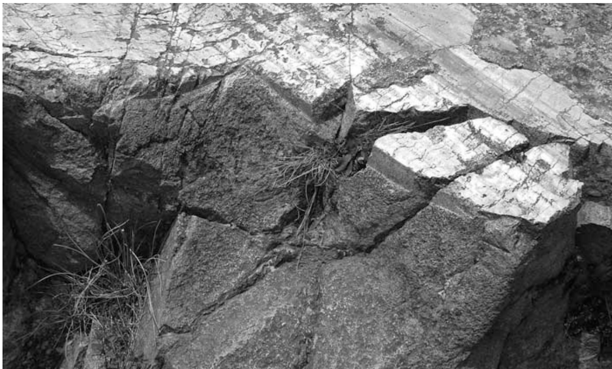
Рис. 30. Следы дисковой пилы в Саксайуамане
