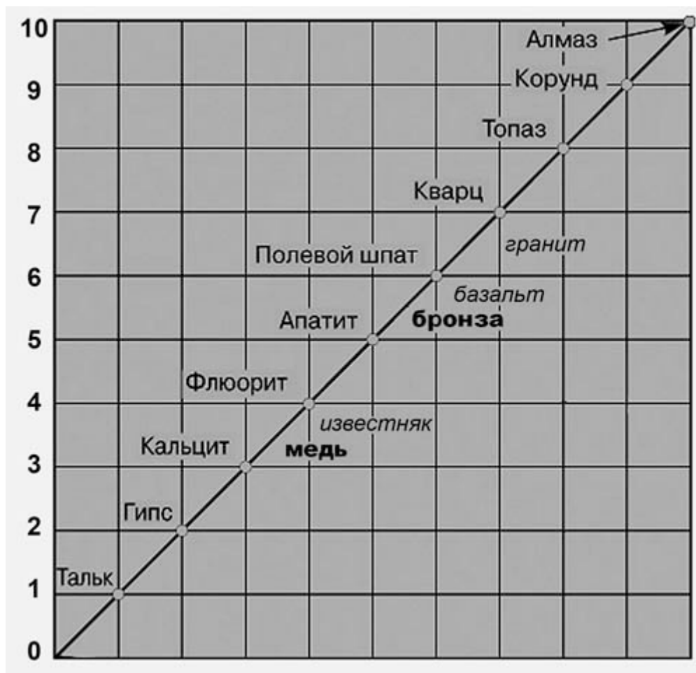
Рис. 13. Шкала Мооса
