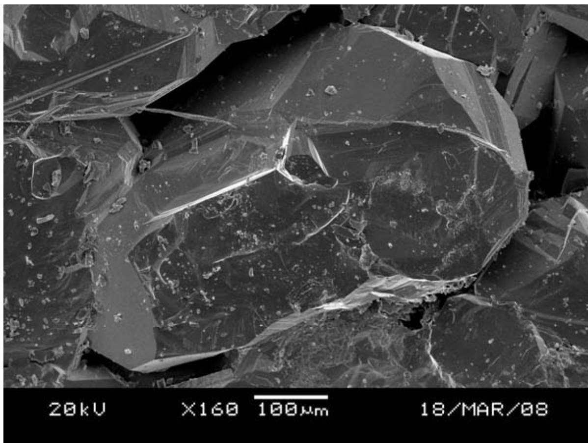
Рис. 36. Сколы кварцевых зерен на образце саркофага под крупным увеличением
