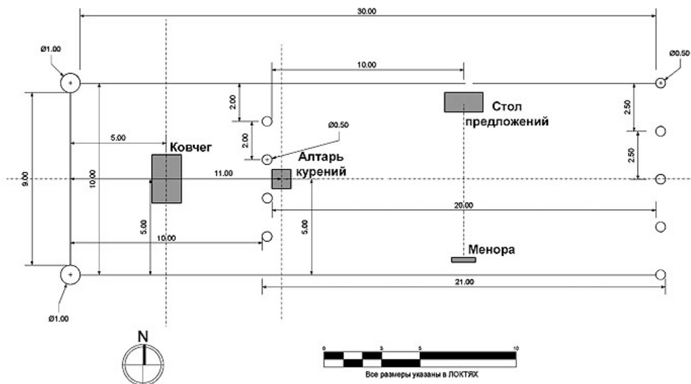
Рис. 199. План Скинии (по Пятикнижию)
